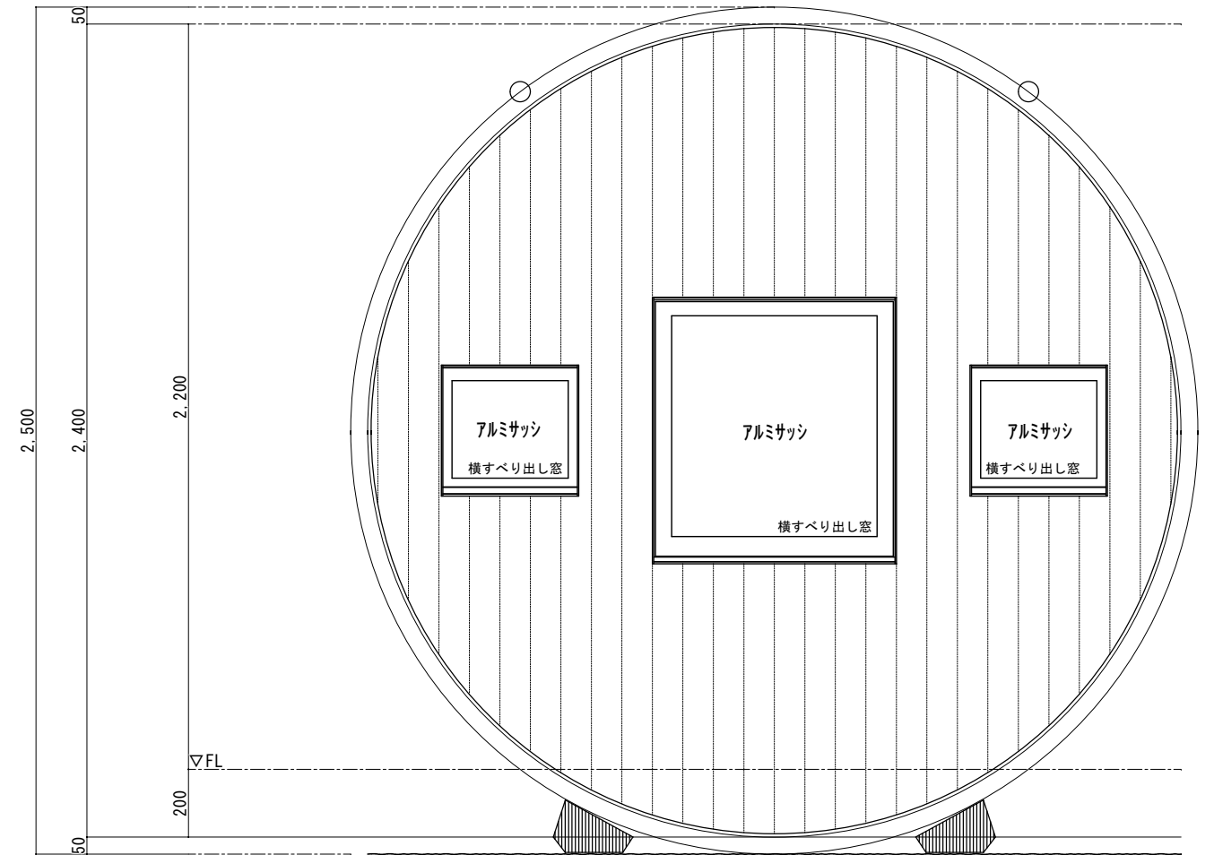
裏側立面図
