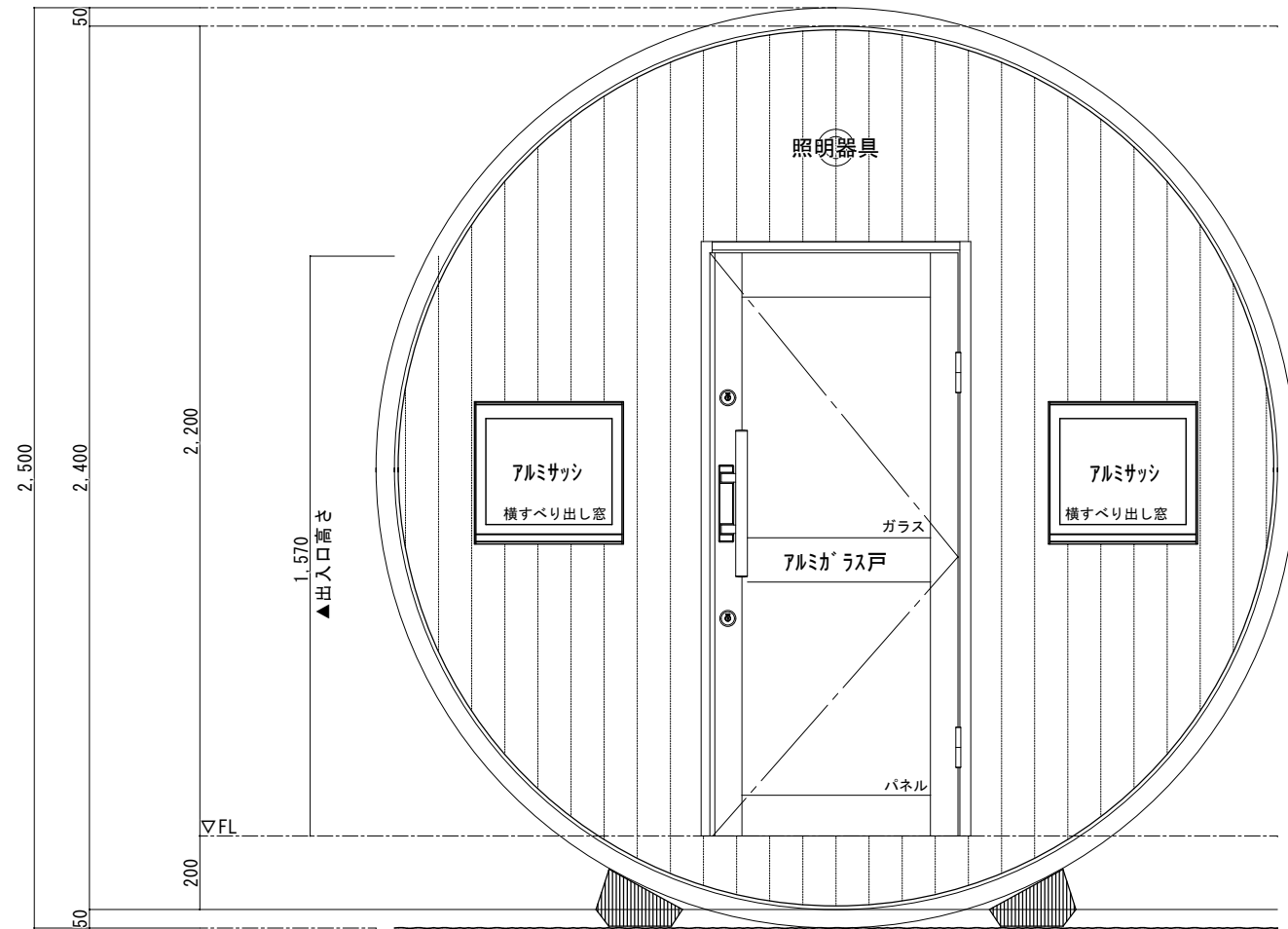
入口側立面図
