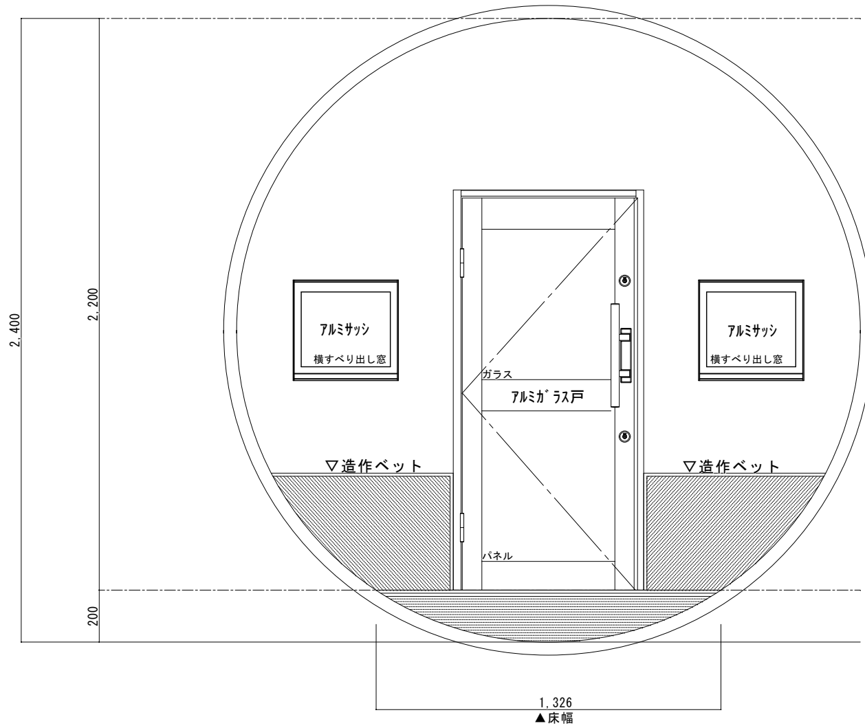
入口側展開図
